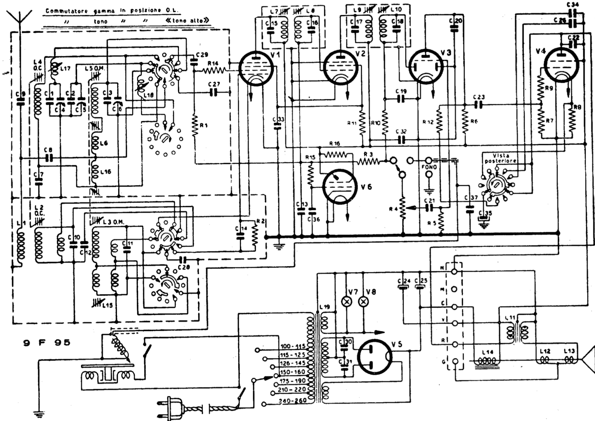
MARELLI - Mod. 9F95 - OL: 145-310 kc; OM: 514-1570 kc; OC1: 5,5-9,7 Mc; OC2: 9,4-16,5 Mc. V1 = 6EA7 (280 V, pl. 90 V sch.) V2 = 6NK7 (idem) V3 = (90 V pl.) V4 = 6L6 (260 V pl. 280 V sch. 12,7 V cat.) V5 = 5Y3 (2 × 350 V) V6 = 6E5. Corr. an. tot. 96 mA, 6L6 72 mA.
